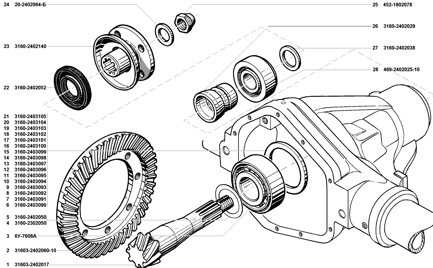
Рис. 54. Передача главная (2302 и 2402)
